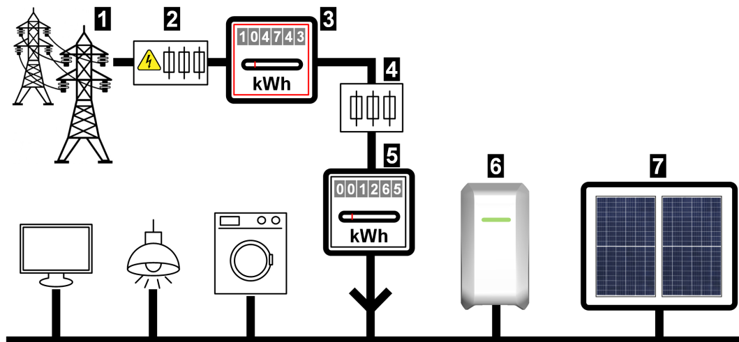
Abb. 14-4: Systemüberblick - Einbindung externer Energiezähler
