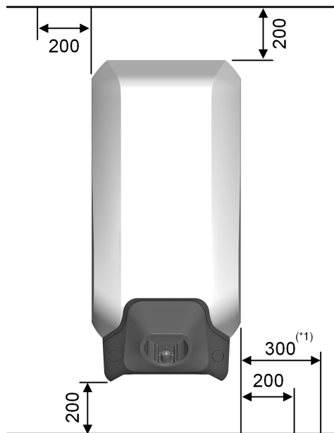
Abb. 8-1: Mindestabstände in Millimeter
