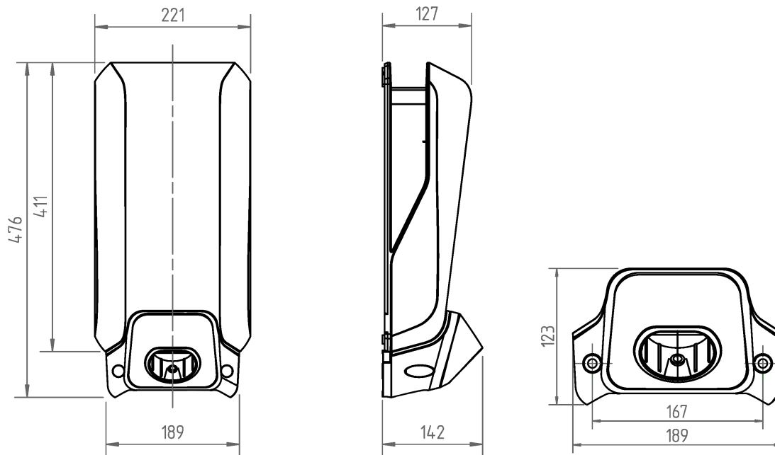
Abb. 21-5: Abmessungen in Millimeter
