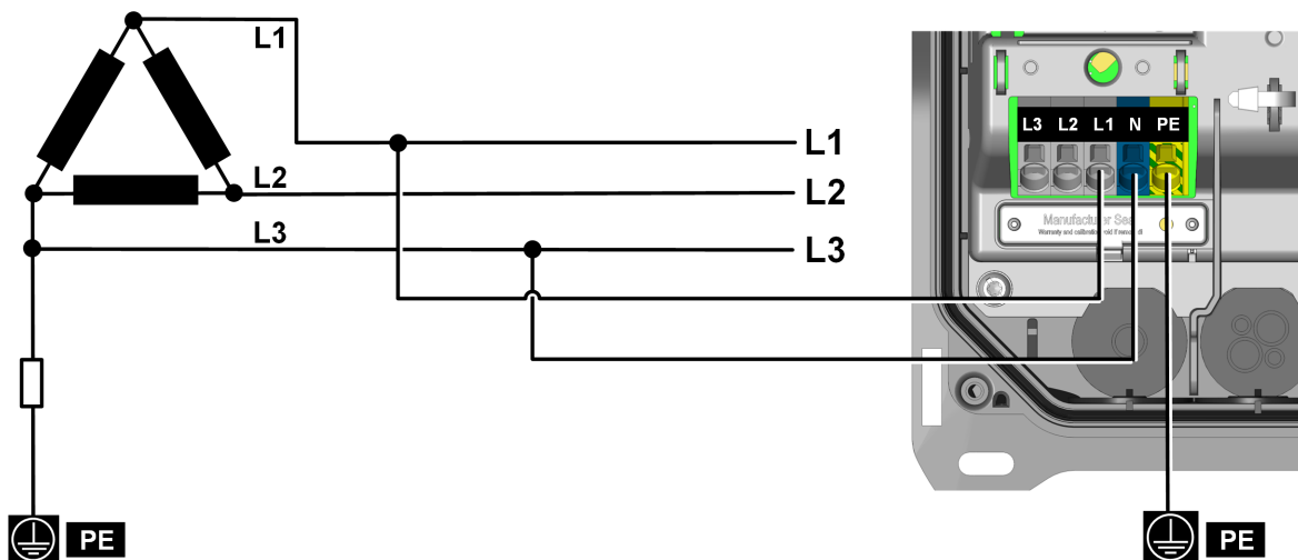
Abb. 9-3: Anschluss an ein Dreileiter-IT-System mit 230 V
