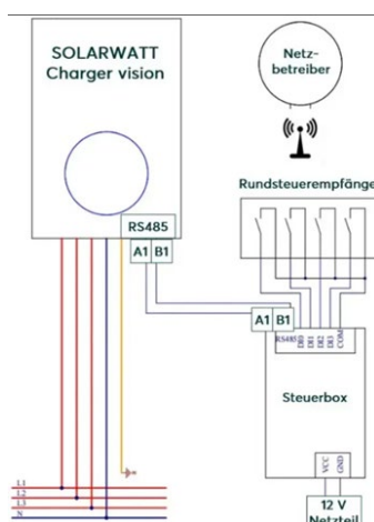
Abb. Anschlussschema
