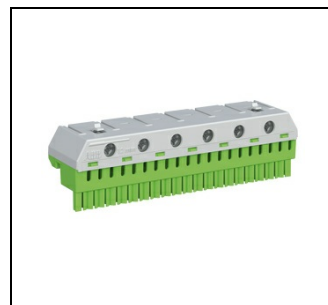
ZK206G PE-Klemmenblock 20x4+6x25qmm EAN Art.-Nr. 2CPX062762R9999 Listenpreis 18,45 €
