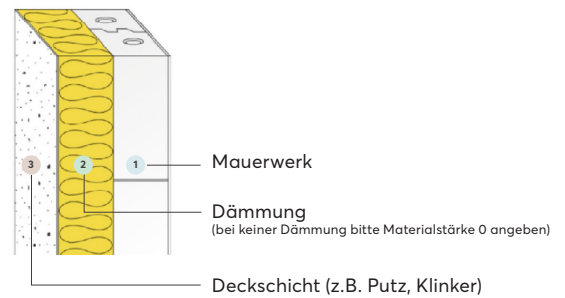
Schnitt Wandaufbau
